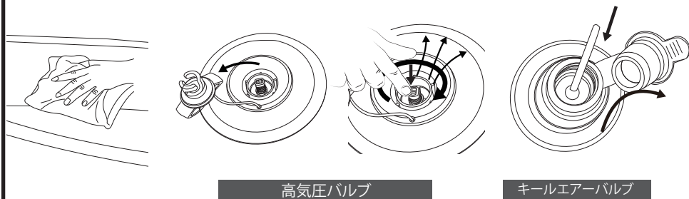
高気圧バルブ
